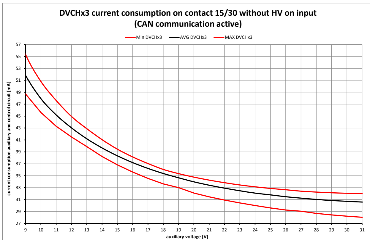
Abbildung 9.2: Stromaufnahme Hilfs- und Steuerstromkreis
