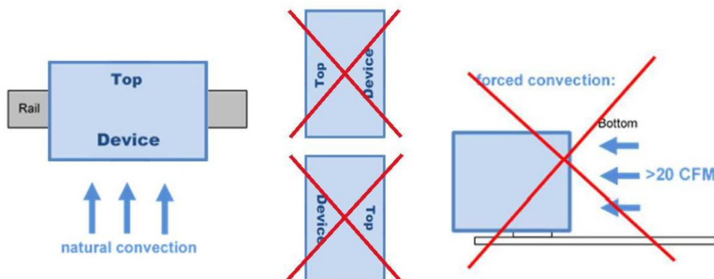
Abbildung 26.3: Montageanleitung: empfohlener Luftstromabstand unten und oben ist 50 mm
