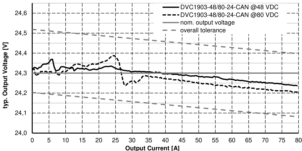
Abbildung 10.3: Typ. Ausgangsspannung in Abhängigkeit des Ausgangsstroms und Gesamttoleranz (0-20 Hz)
