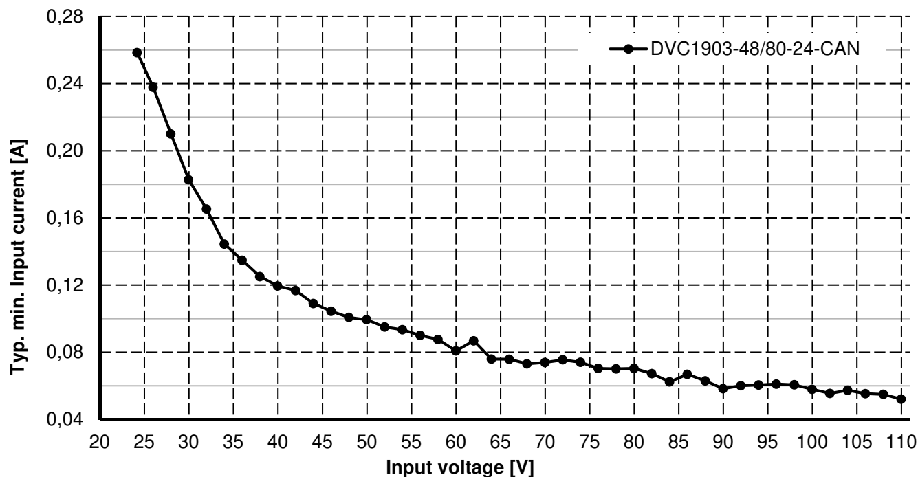
Abbildung 10.2: Leerlaufstromaufnahme
