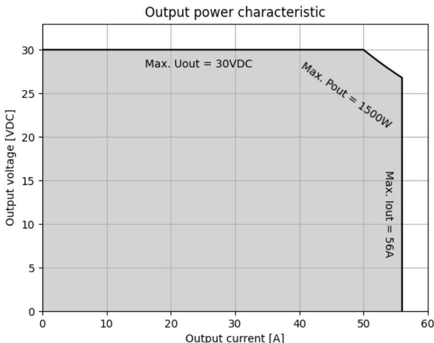
Abbildung 9.1: Ausgangsleistung DVCH1503-700-24
