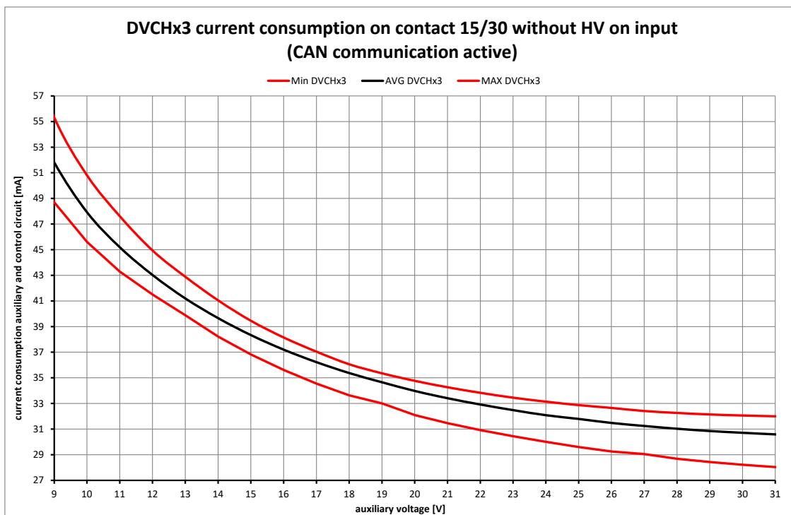
Abbildung 9.3: Stromaufnahme Hilfs- und Steuerstromkreis
