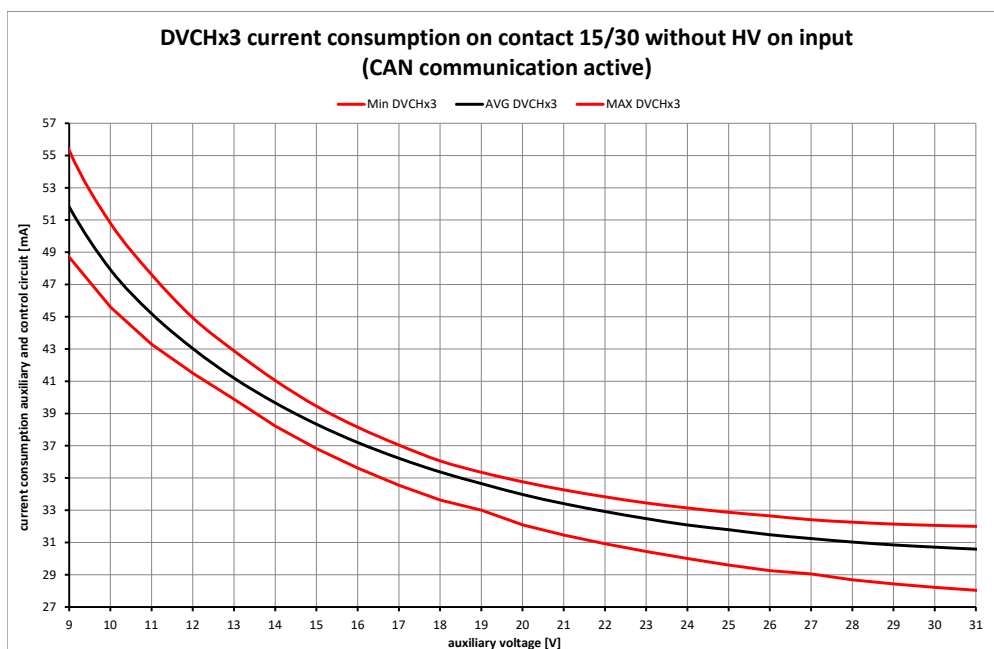
Abbildung 9.4: Stromaufnahme Hilfs- und Steuerstromkreis
