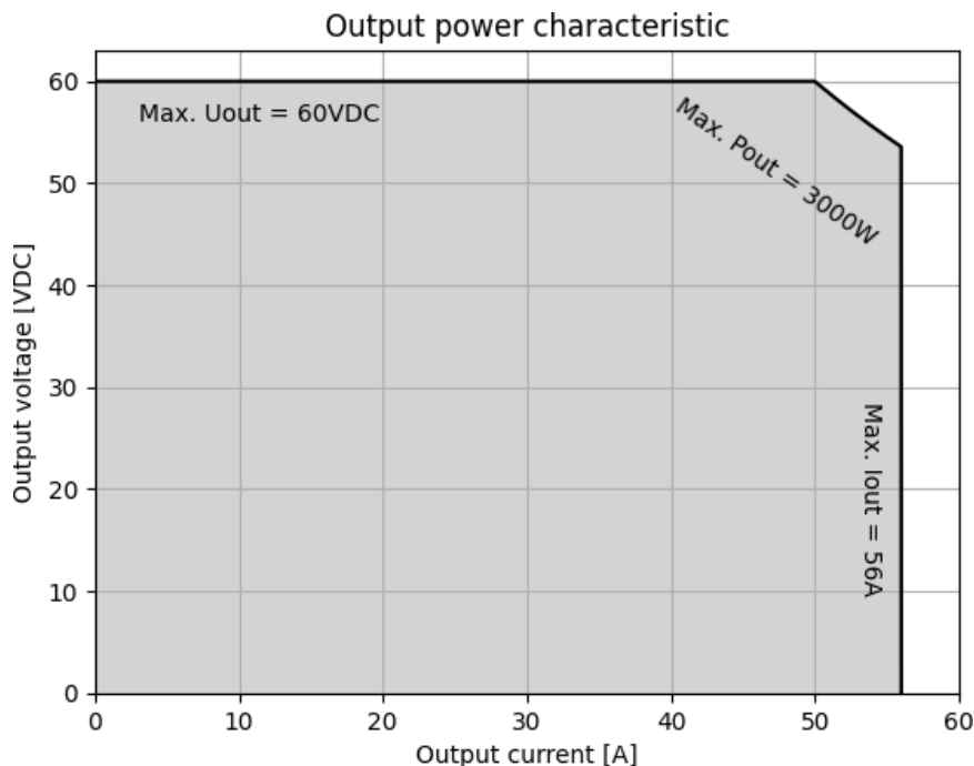
Abbildung 9.3: Ausgangsleistung DVCH3003-400-48
