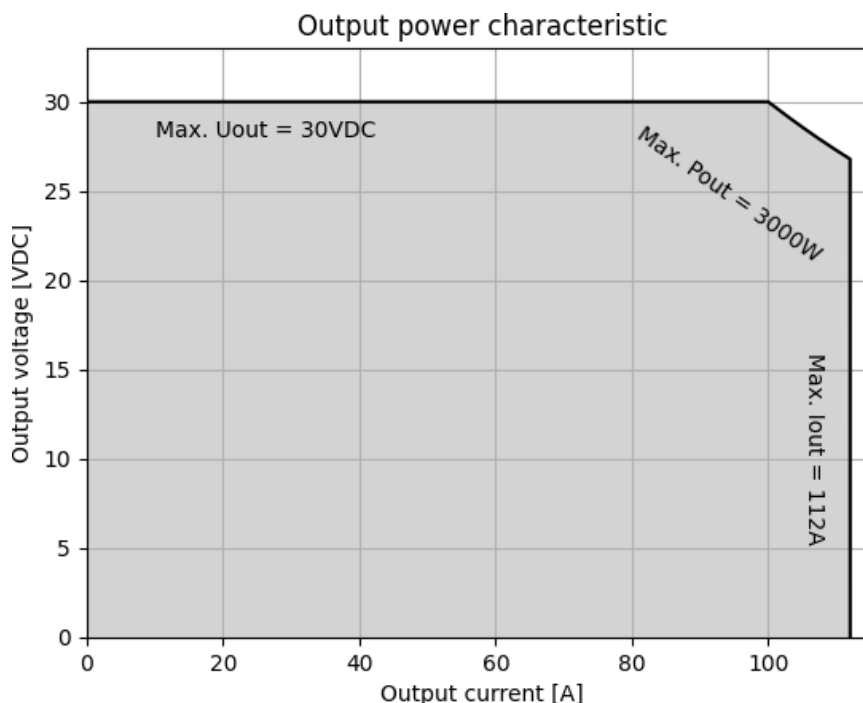
Abbildung 9.2: Ausgangsleistung DVCH3003-400-24
