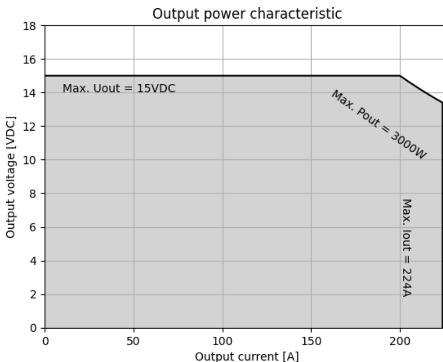
Abbildung 9.1: Ausgangsleistung DVCH3003-400-12
