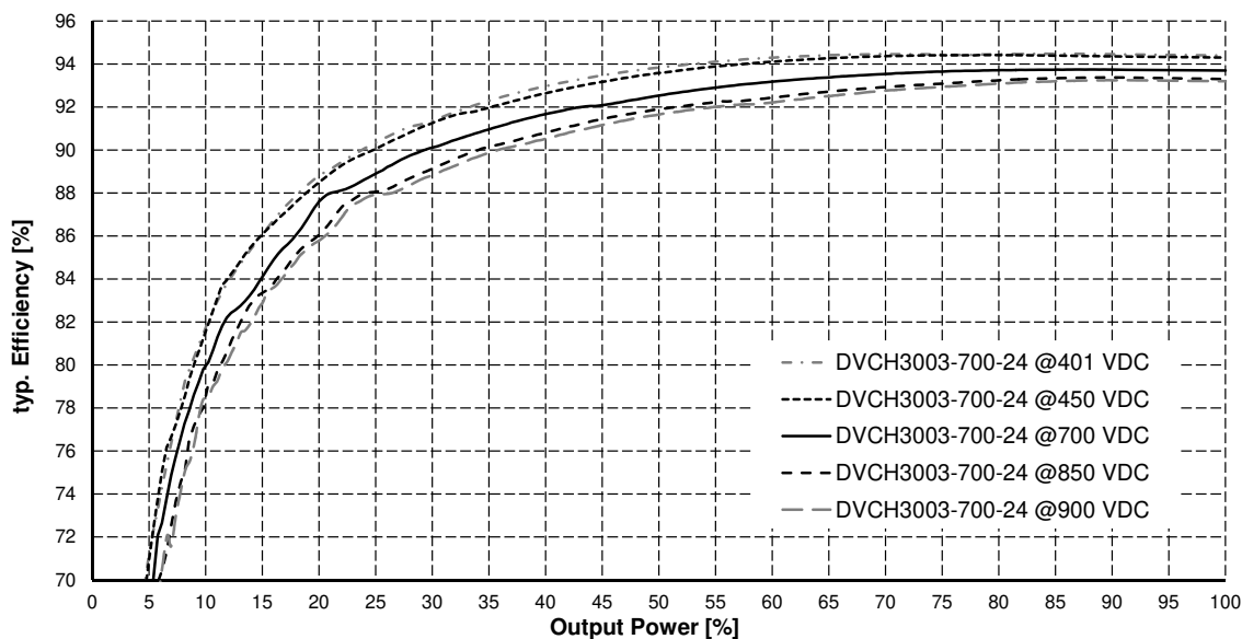
Abbildung 9.4: Wirkungsgrad in Abhängigkeit der Ausgangsleistung
