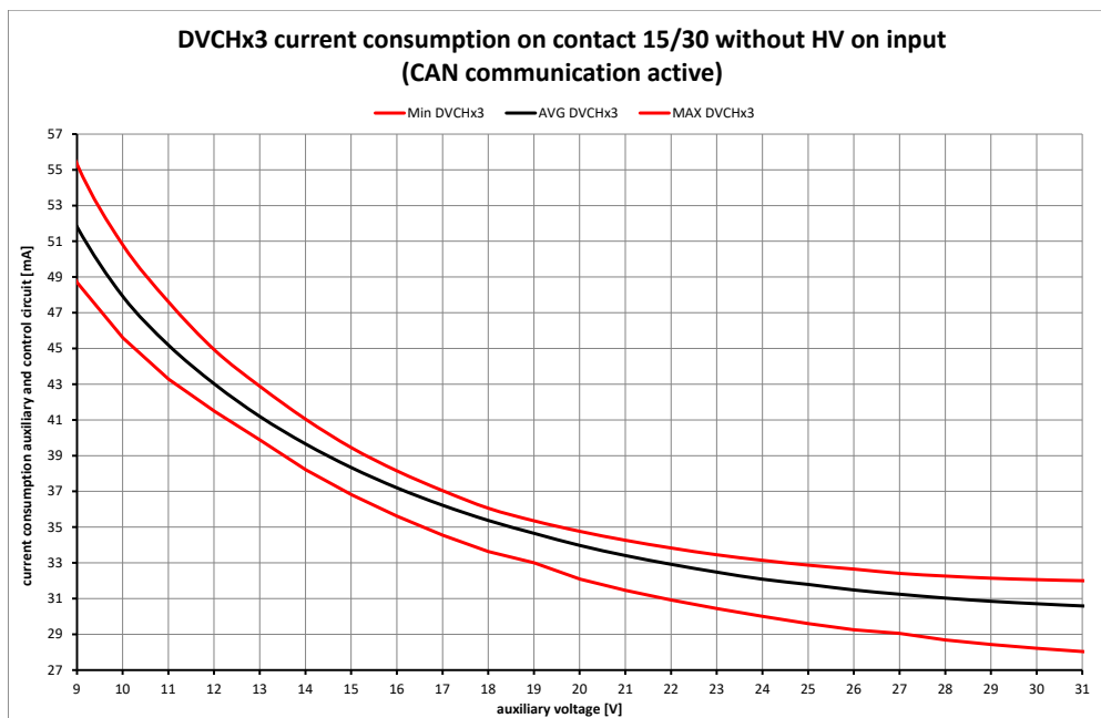
Abbildung 9.5: Stromaufnahme Hilfs- und Steuerstromkreis
