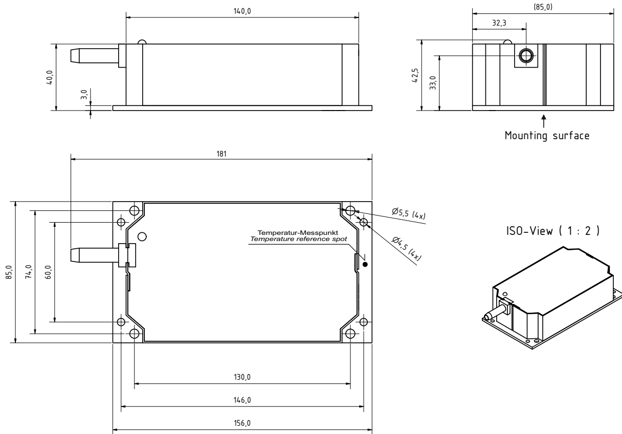
Abbildung 8.1: Abmessungen
