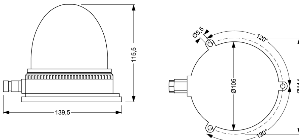
Abbildung 3.1: Abmessungen
